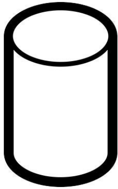
원통 (Cylinder)
