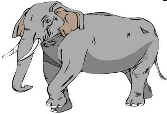
코끼리 (Elephant)
