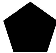
오각형 (Pentagon)
